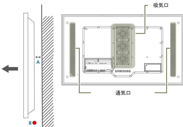
図 1.1 側面図
