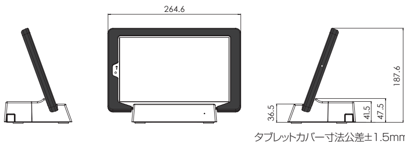
タブレットカバー寸法公差±1.5mm
